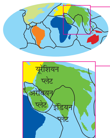
चित्र 15.10 : पृथ्वी की प्लेट।
