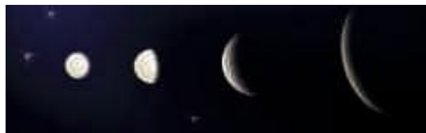
चित्र 17.20 : शुक्र की कलाएँ।
