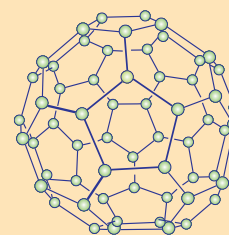
C-60 बकमिस्टरफुलेरीन की संरचना
